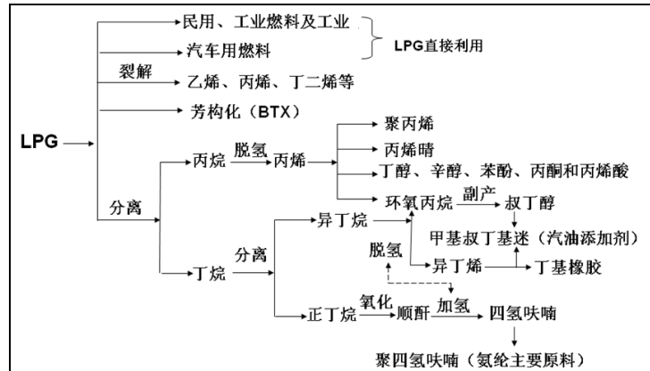
图 1 LPG 产业链示意图
